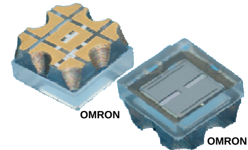
RF MEMSスイッチ
